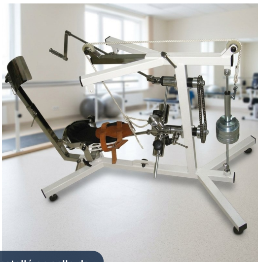
Appareil de rééducation de la cheville installé en salle de
